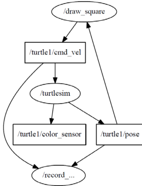
图 9.1 rosvim 记录运行时的节点和话题的计算图。
