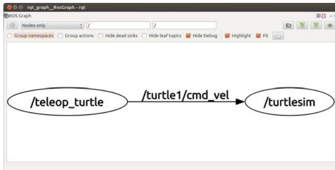
图 2.2 rqt_graph 界面，展示了 turtlesim 例子中的节点图结构。其中省略了调试节点，包括 rosout 节点。
